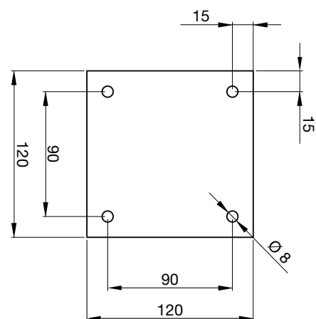
Hålbild för samtliga konsoler/fästen
