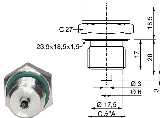
Typ 1: G \frac{1}{2} "A, skyddat membran
